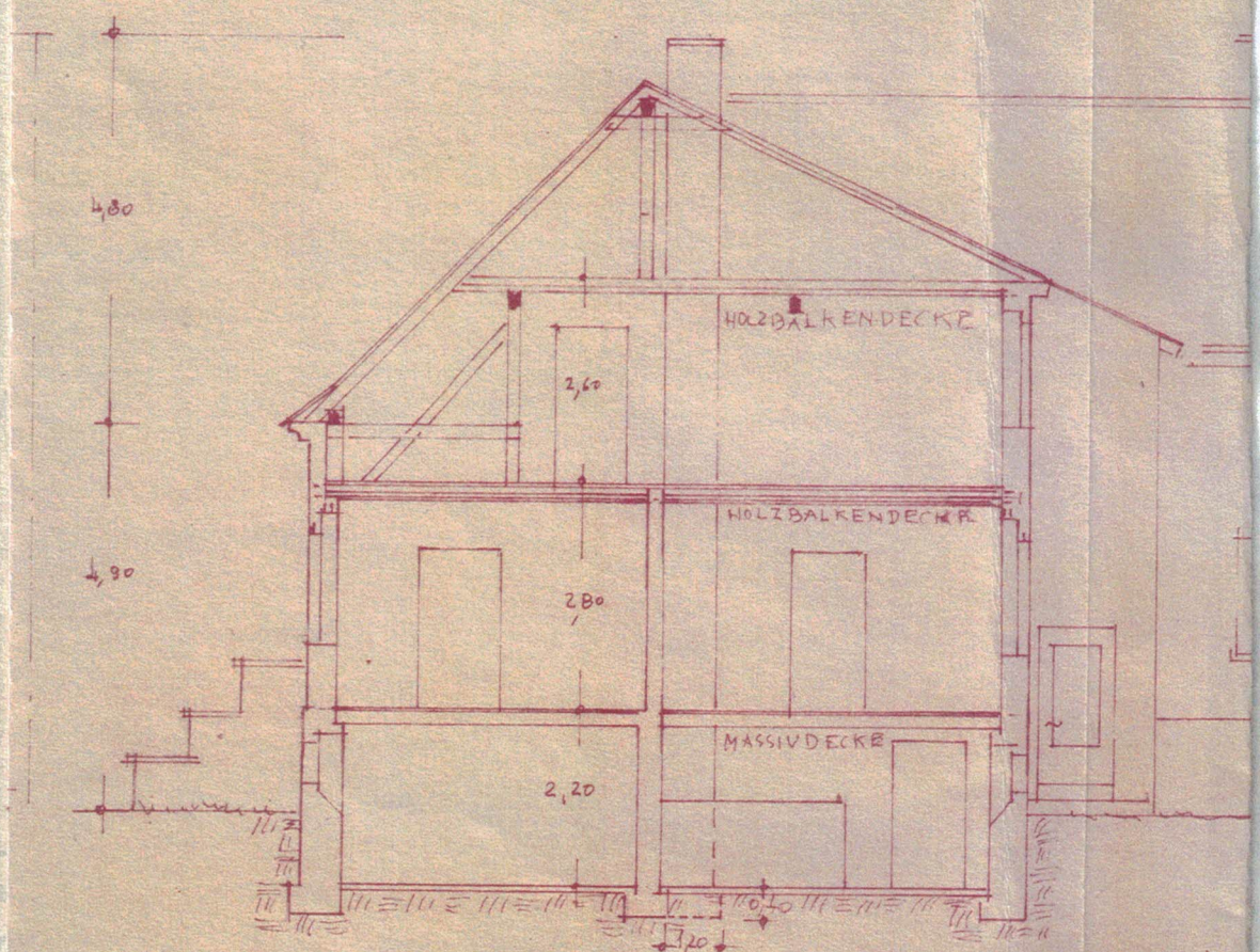
SCHNITT A-B
