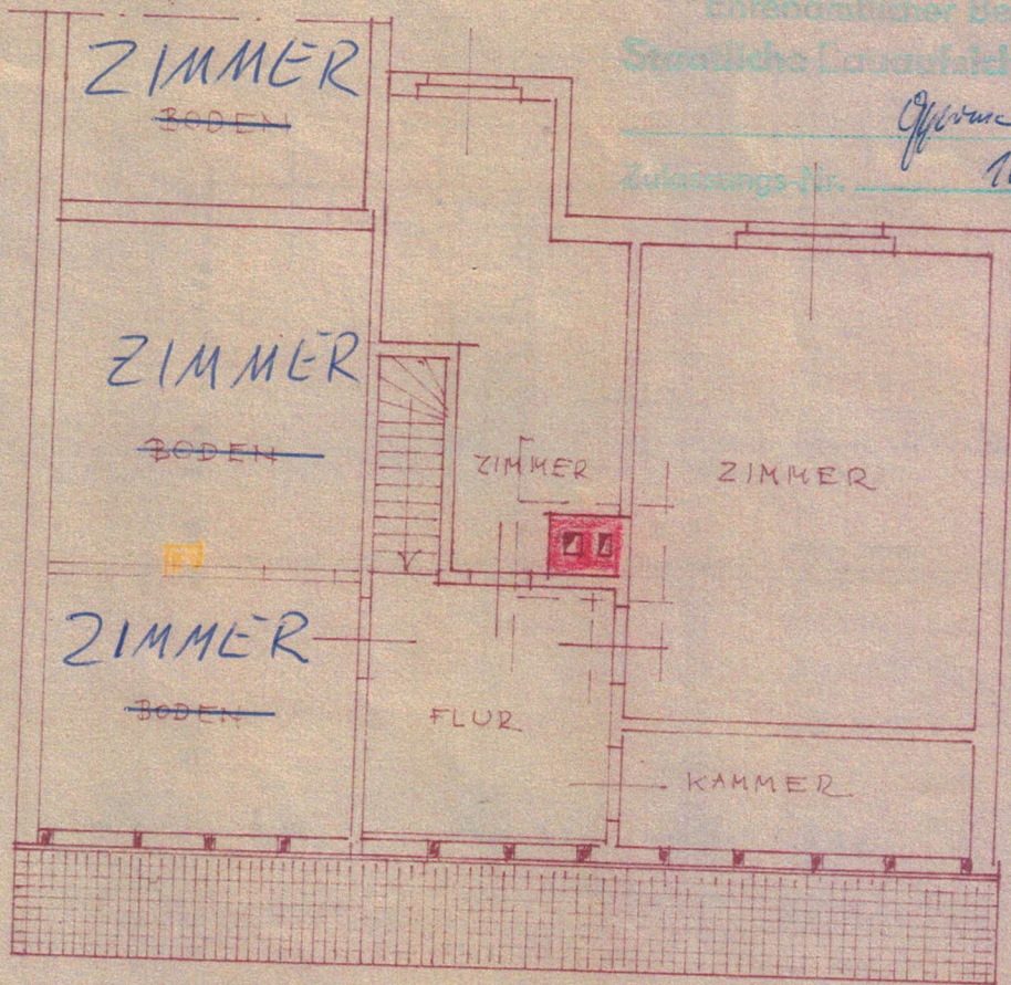
DACHGESCHOSS
