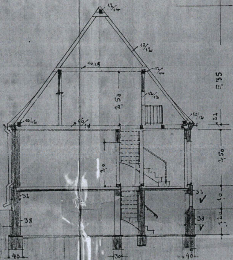
Schnitt A-B.
